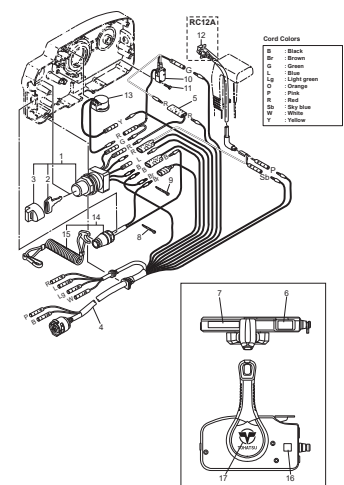
Fig.18 COMPONENT PARTS OF REMOTE CONTROL (ELECTRIC PARTS) リモコンボックス構成部品(電気部品関係)
