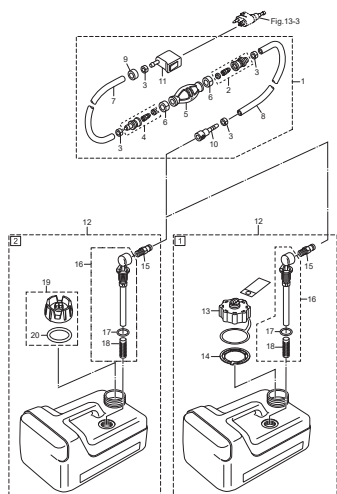
Fig.16 FUEL TANK フエルトンク
