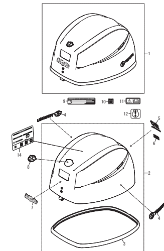
Fig. 16 TOP COWL トップカウル
