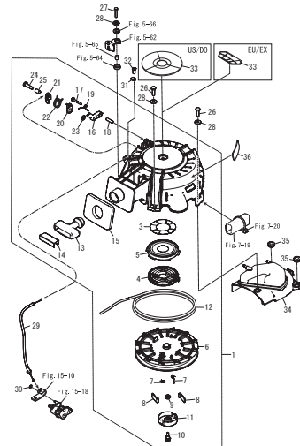
Fig. 6 RECOIL STARTER リコイルスタータ
