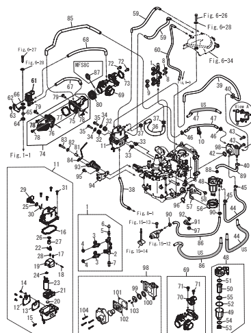
Fig. 5 INTAKE MANIFOLD · FUEL PUMP インテークマニホールド・フェエルポンプ
