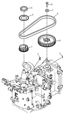
Fig. 4 PULLEY · TIMING BELT プーリー・タイミングベルト
