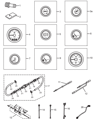
Fig. 22 RIGGING KIT (1) リギングキット (1)
