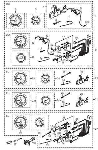
Fig. 22 RIGGING KIT (1) リギングキット (1)
