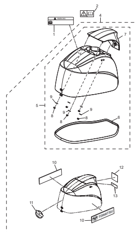
Fig.18 TOP COWL トップカウル
