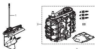
Fig. 26 ASSEMBLY · KIT PARTS アッセンブリ・キットパーツ
