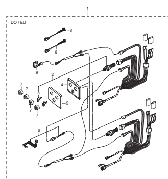
Fig. 25A RIGGING KIT (2) リギングキット (2)
