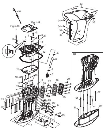
Fig.13 BRACKET ブラケット
