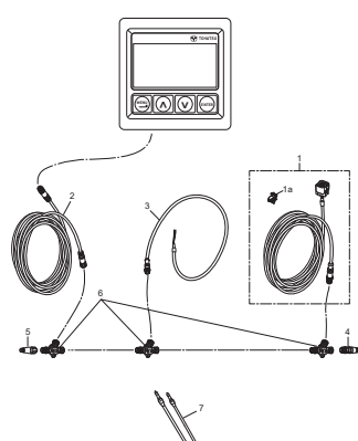
Fig. 25A RIGGING KIT (2) リギングキット (2)
