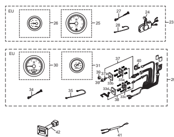
Fig. 25 RIGGING KIT (1) リギングキット (1)
