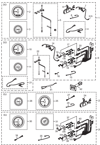
Fig. 25 RIGGING KIT (1) リギングキット (1)
