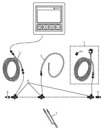
Fig. 25A RIGGING KIT (2) リギングキット (2)
