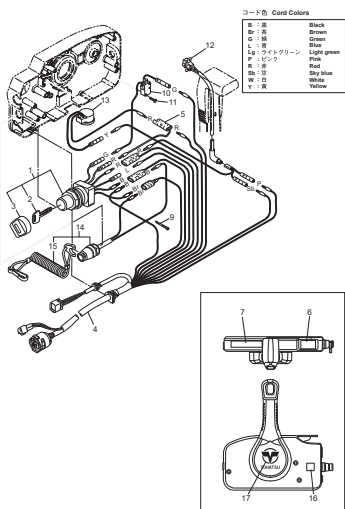
Fig. 24 OPTIONAL PARTS (2) オプショナルパーツ (2)
