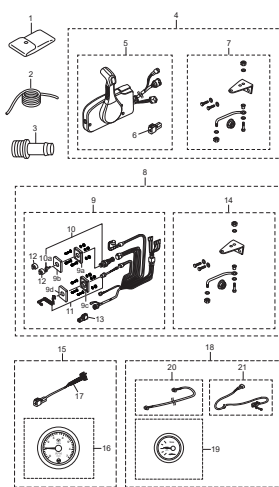
Fig. 26 ACCESSORIES • RIGGING KIT アクセサリ・リギングキット
