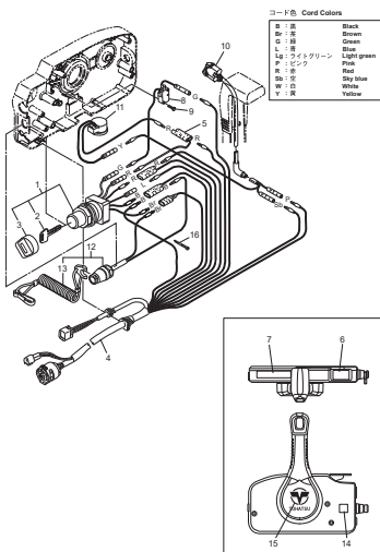
Fig. 25 COMPONENT PARTS OF REMOTE CONTROL (ELECTRIC PARTS) リモコンボックス構成部品 (電装品関係)
