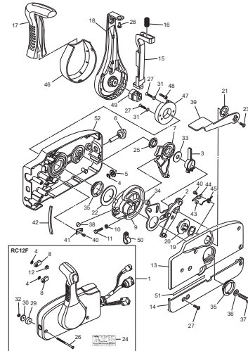
Fig. 27 REMOTE CONTROL • REMOTE CONTROL PARTS リモートコントロール・リモートコントロールパーツ
